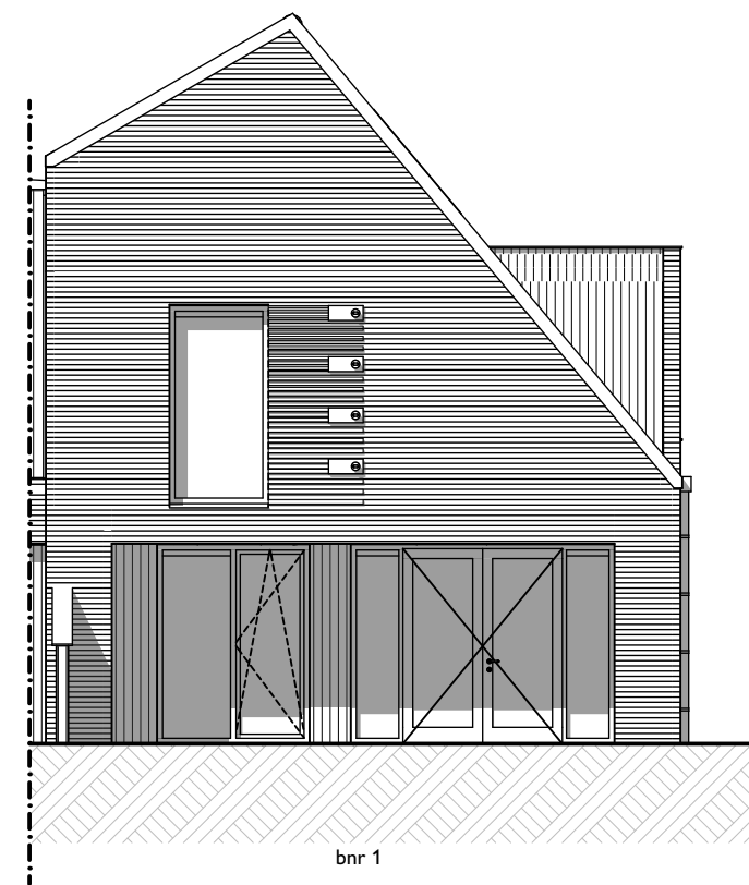
Achtergevel
