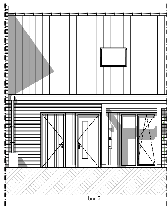
Voorgevel
