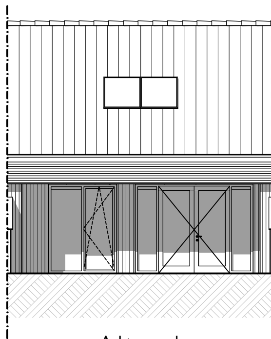
Achtergevel
