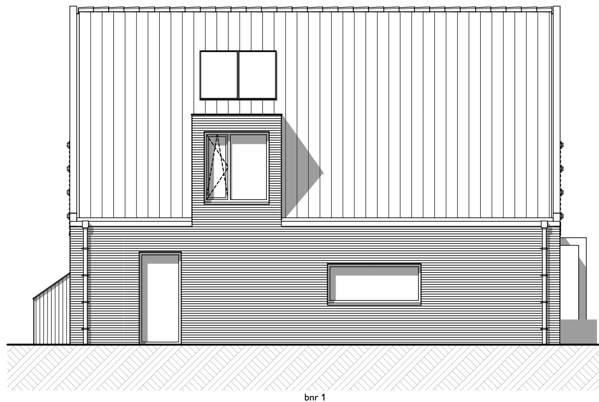
Linkergevel
