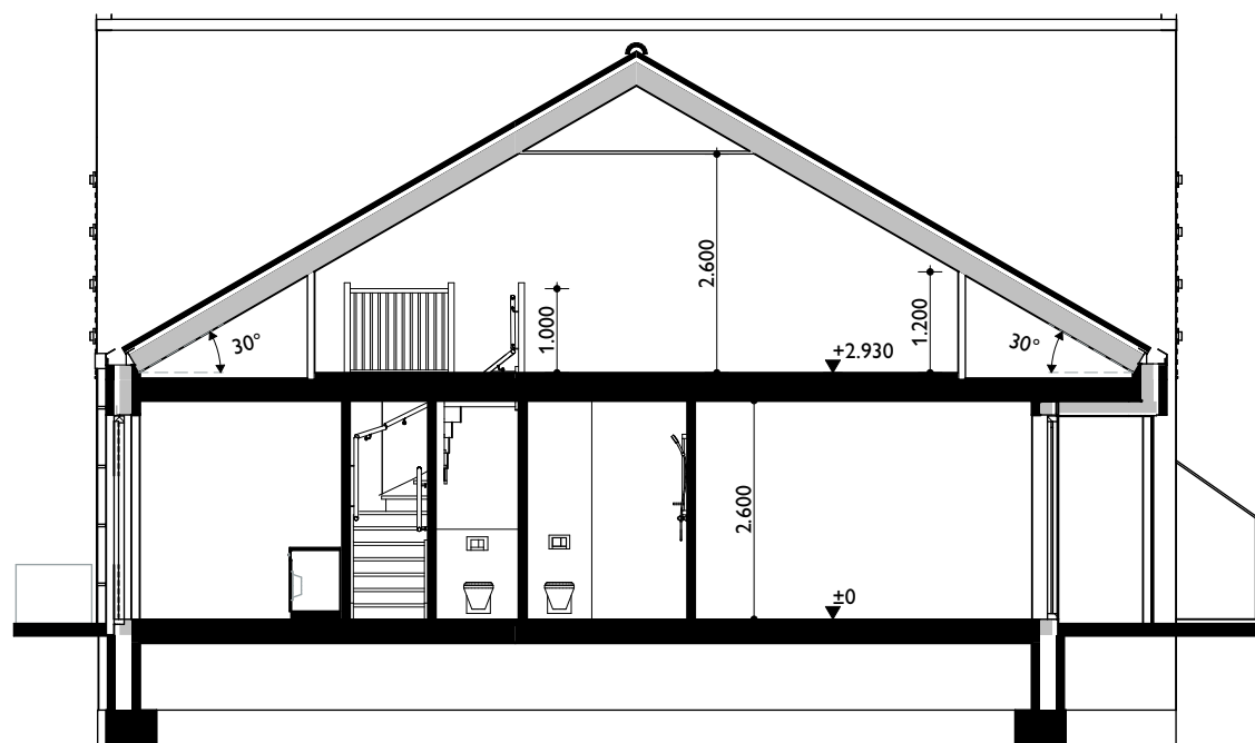
Doorsnede
