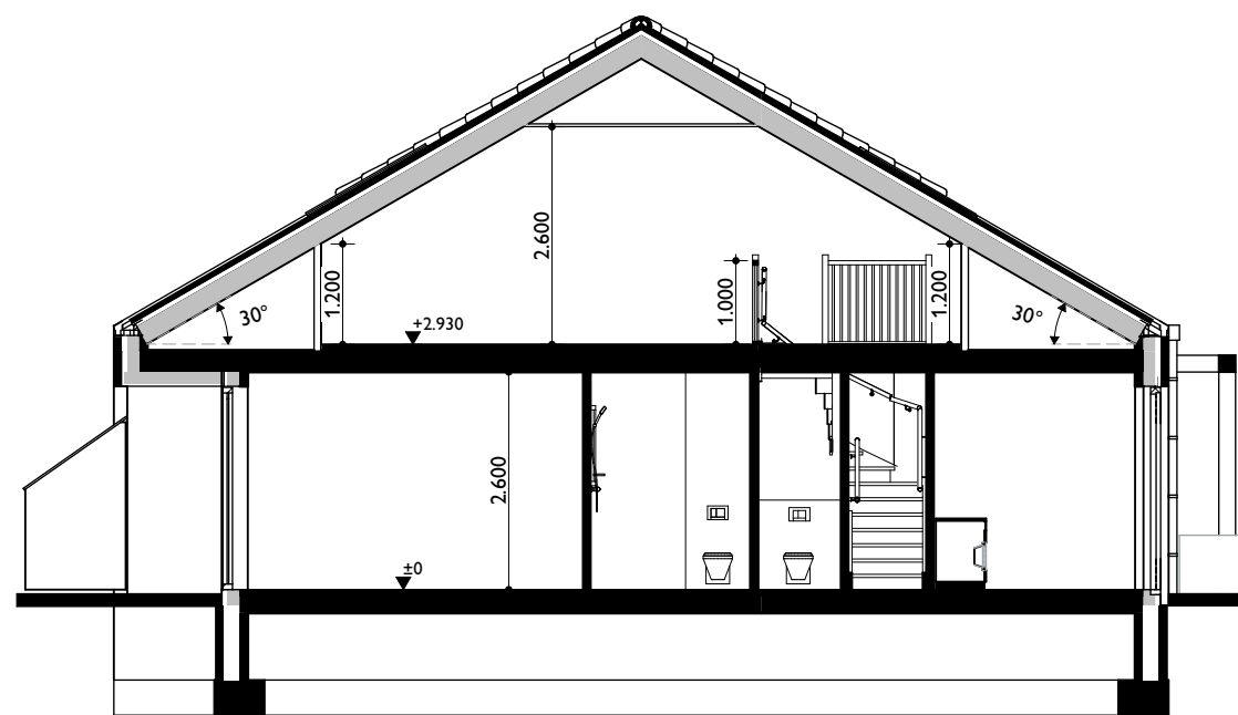
Doorsnede
