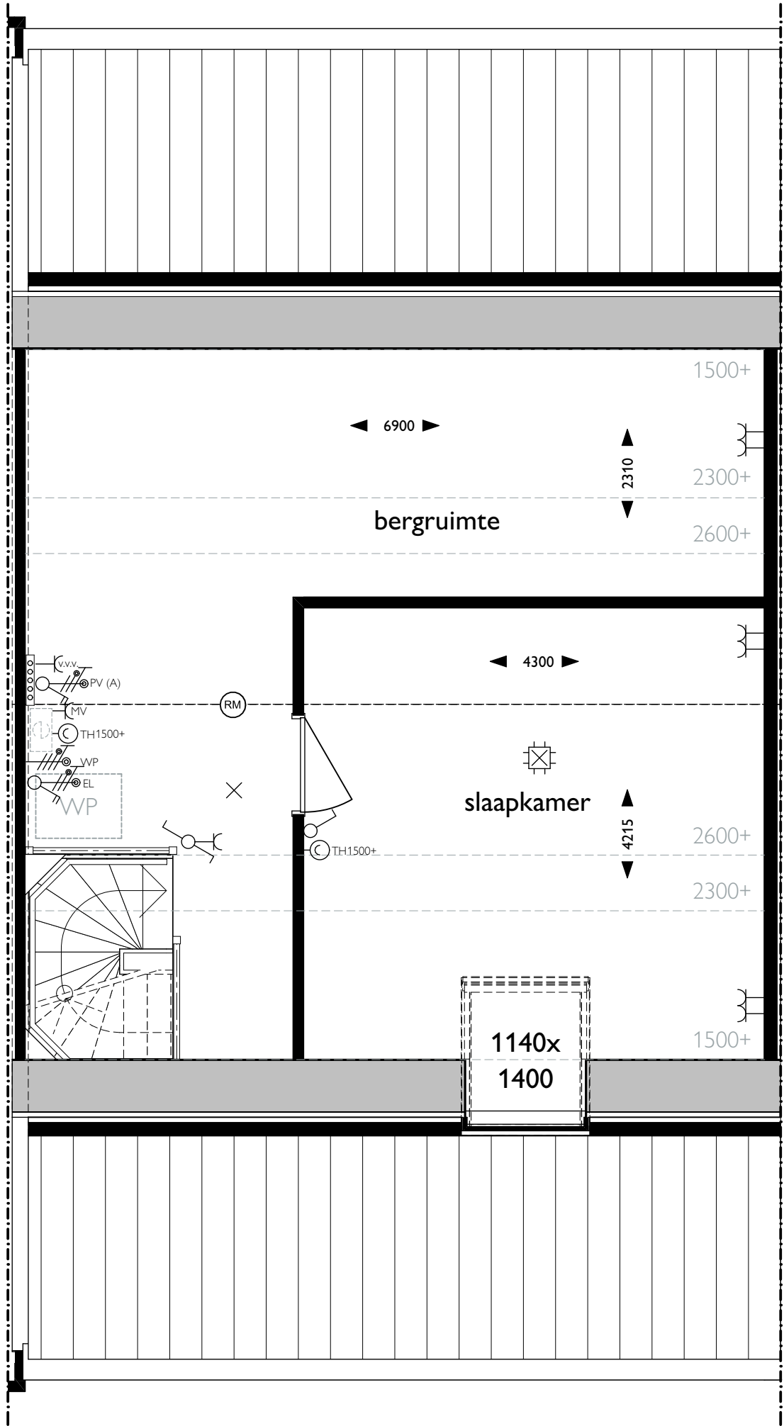
01 eerste verdieping
