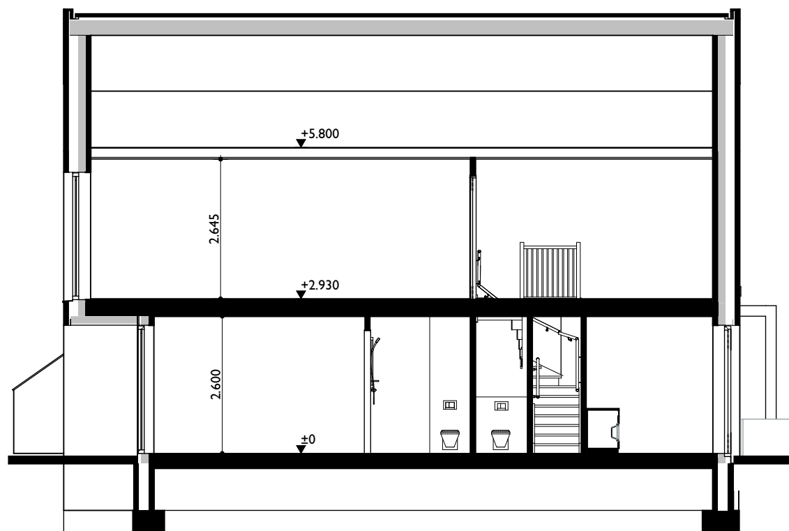
Doorsnede
