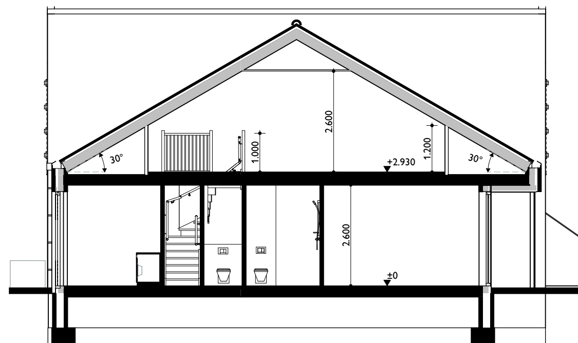
Doorsnede
