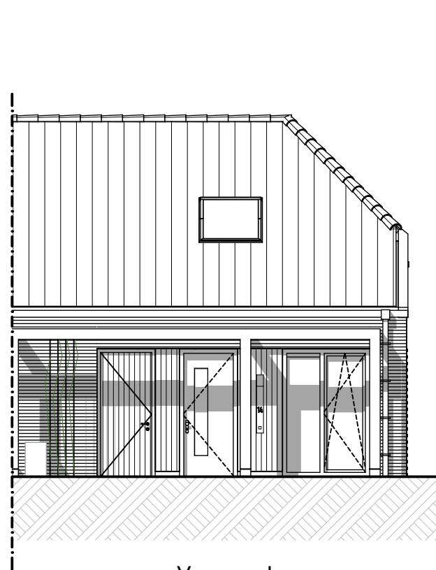
Voorgevel
