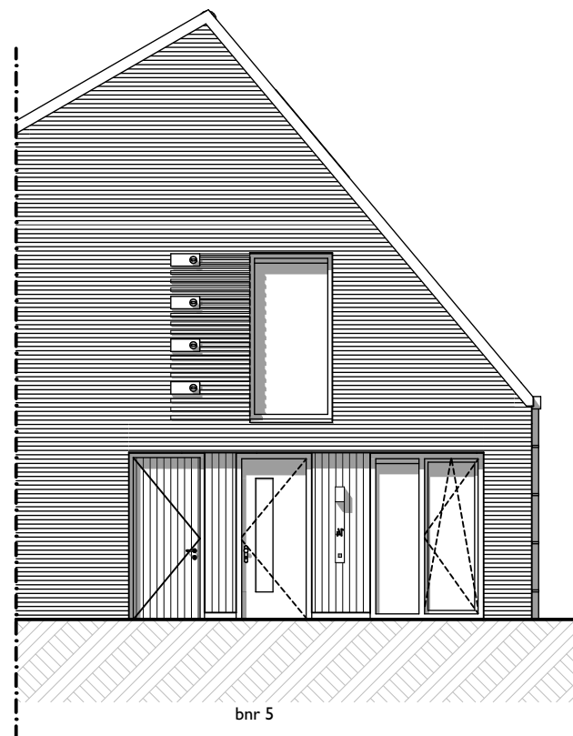
Voorgevel
