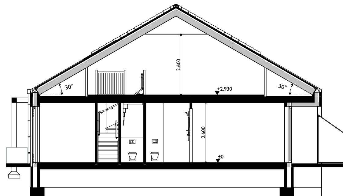
Doorsnede
