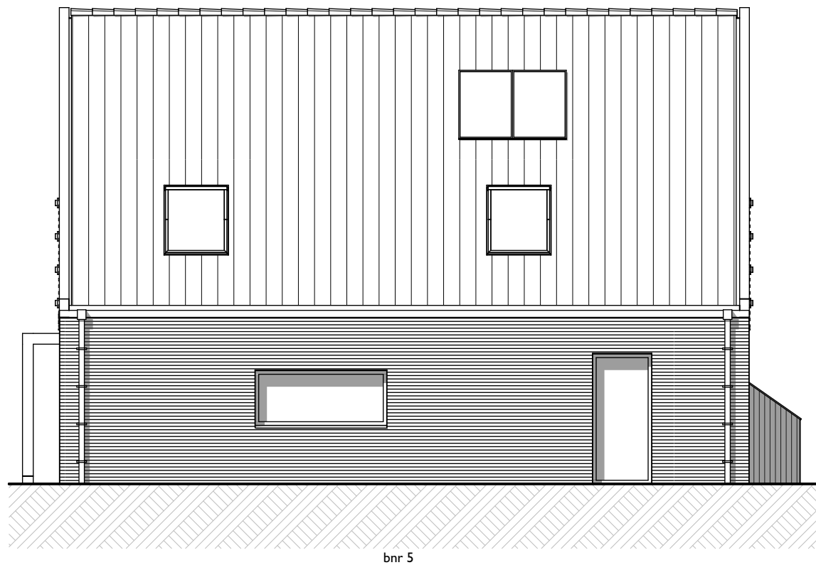
Rechtergevel
