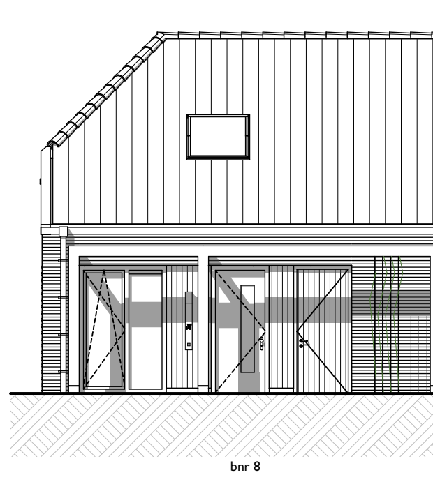
Vorgevel
