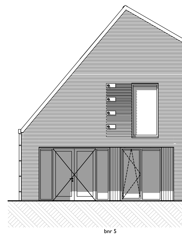
Achtergevel
