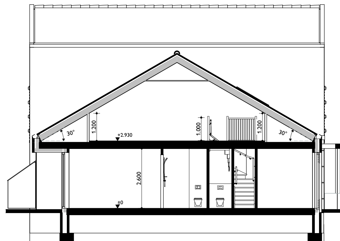
Doorsnede
