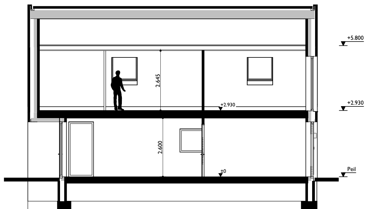
Doorsnede
