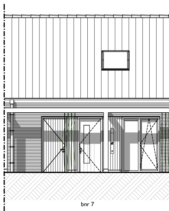
Voorgevel
