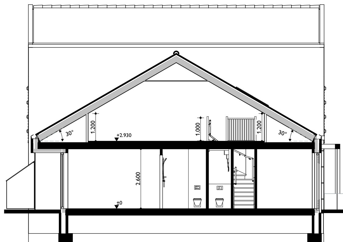
Doorsnede
